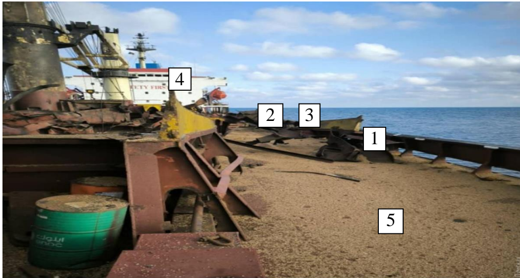
Рис. 1. Вид руйнування ракетною вантажних трюмів з фумігованим фосфіном зерном та вибуховим викидом горілого зерна балкера «АУА» (1- відірвані частини комінгсу, 2- покручені частини кришок трюмів, 3- викид частини секції кришки трюму, 4- вибите вибухом скло надбудови, 5- викид з трюмів горілого зерна на вантажні палуби лівого борту)
